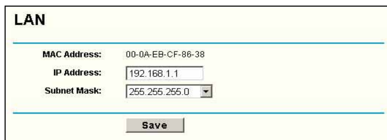
Figure 5-3 LAN
